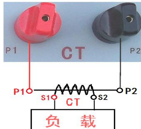
图 17、CT 一次通流接线图
