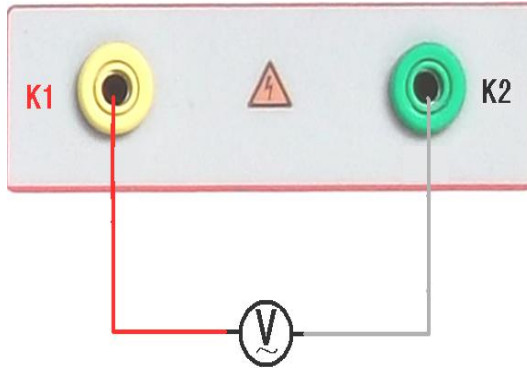
图 36, 电压校准接线图
