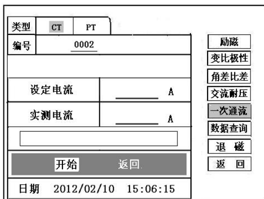
图 16、CT 一次通流测试界面
