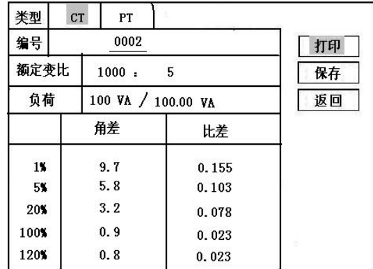
图 15, CT 角差比差测试结果界面
