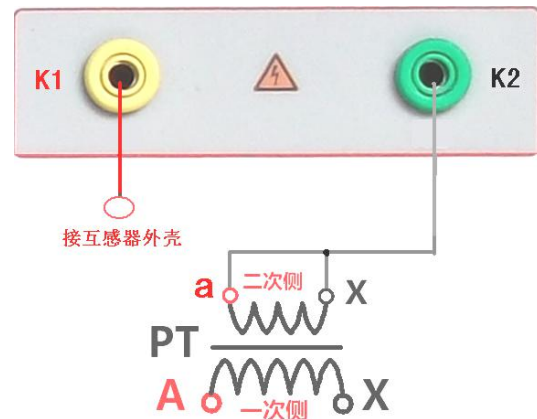
图 28, PT 交流耐压接线图
