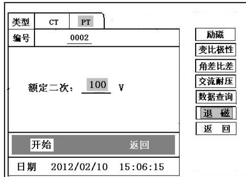
图 22, PT 退磁界面
