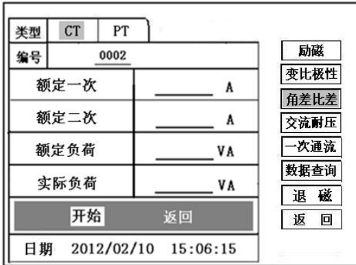
图 14 , CT 角差比差测试界面
